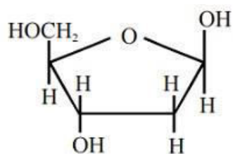
\beta -D-2deoxyribose
